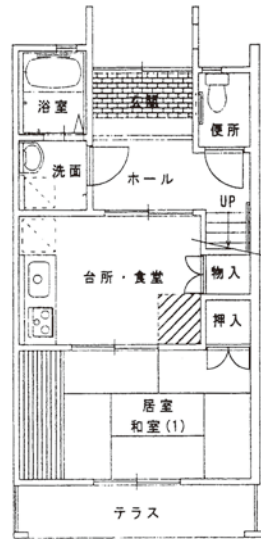
1階平面図
